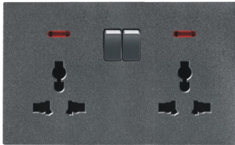
型號： 2KZ13/N $200.00 146型雙多功能三插帶開關 帶LED指示燈 包裝數量： 5只 / 盒 50只 / 箱
