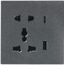
型號： SZ12Z13USB $330.00 二極帶三極多功能通用插座 +USB+Type-c 包裝數量： 10只 / 盒 100只 / 箱
