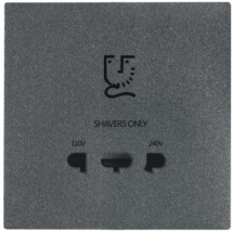
型號： S-GX $650.00 刮鬚插座 包裝數量： 7只 / 盒 70只 / 箱
